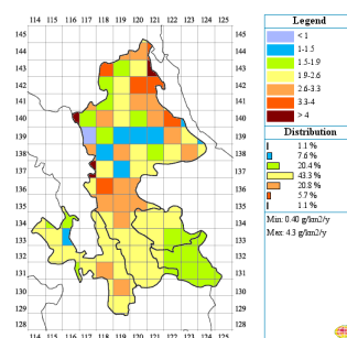
Рисунок 1. Карты суммарных выпадений СОЗ и концентраций в воздухе в стране в 2011 г.
