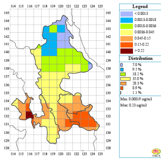
Пространственное распределение Б[а]П концентрации в воздухе, нг/м 3
