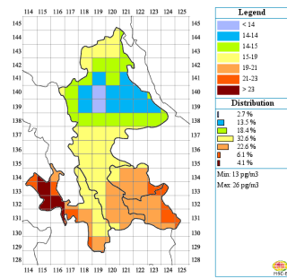
Пространственное распределение ГХБ концентрации в воздухе, пг/м 3
