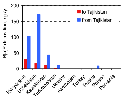
Рисунок 2. Антропогенные выпадения от 10 основных вкладчиков на страну и антропогенные выпадения от Таджикистана на эти страны в 2011 г.
