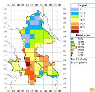
Суммарные выпадения Cd, г/км²/год
