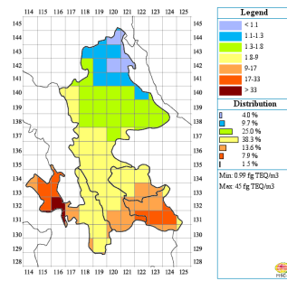
Пространственное распределение ПХДД/Ф концентрации в воздухе, фг ТЭ/м 3
