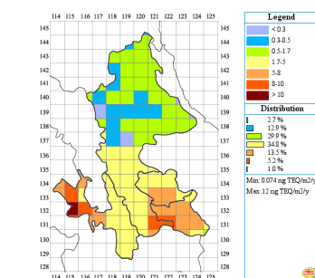
Рисунок 1. Карты суммарных выпадений СОЗ и концентраций в воздухе в стране в 2011 г.
