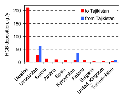
Рисунок 2. Антропогенные выпадения от 10 основных вкладчиков на страну и антропогенные выпадения от Таджикистана на эти страны в 2011 г.
