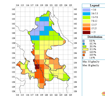
Суммарные выпадения Hg, г/км²/год
