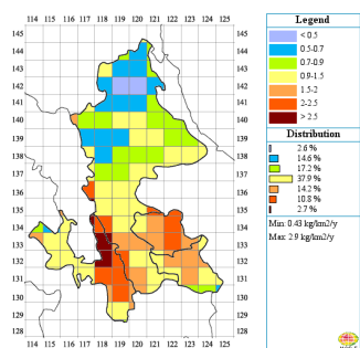
Суммарные выпадения Pb, кг/км²/год
